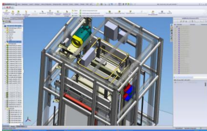
SolidWorks Ansicht eines Glasaufzuges, der in der Eingangshalle des neuen Technologiecenters in Scheibbs/Österreich zu finden ist.
